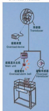
超载保护器 Overload Protector
