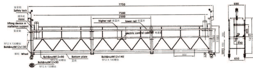
ZLP800型工作平台 ZLP800 type working platform
